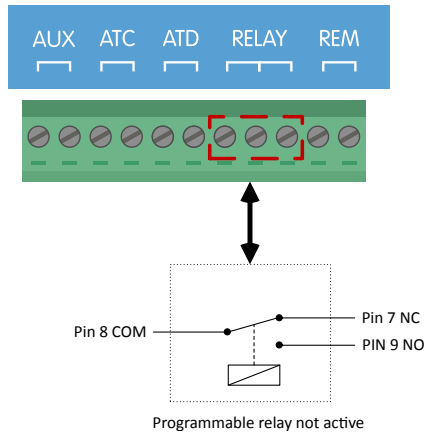
Aansluitingen voor het programmeerbare relais
