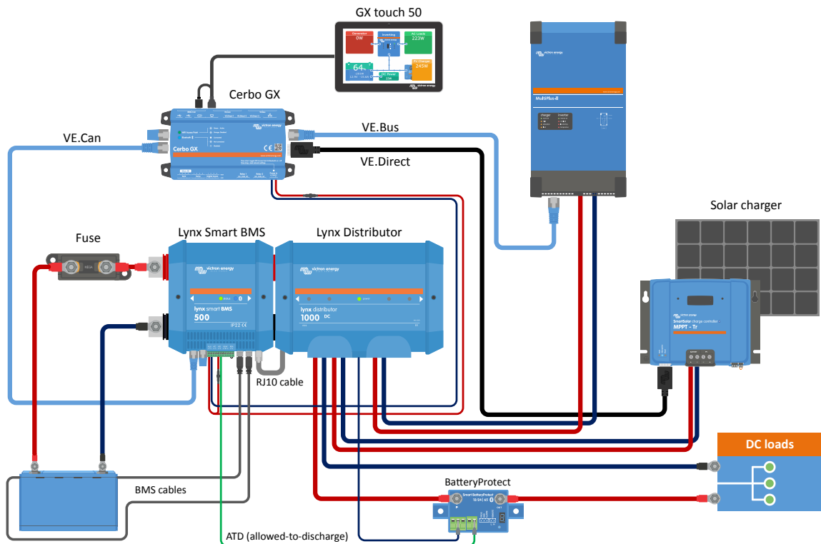
System met een Lynx Smart BMS en een enkele Lynx Distributor
